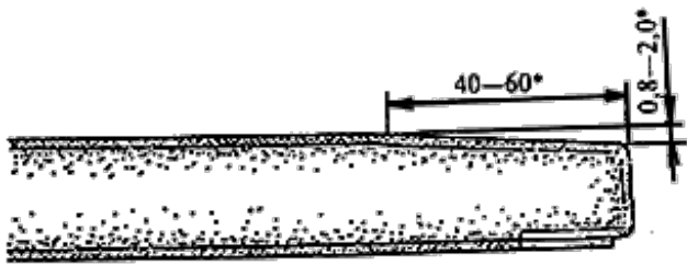
Рисунок 2 - Утоненная с лицевой стороны кромка (УК)
